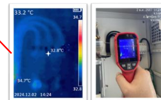
ฟาส MCCB 32.8 °C
