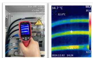
สําม MCCB 35.0 °C
