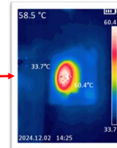
RTU FAN 60.4 °C พัดลมทำงานปกติ
