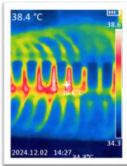
ภายในตู้ DC Panal Box อุณหภูมิ 38.6 °C
